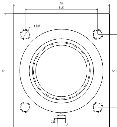
DGS1-1磁性开关槽
